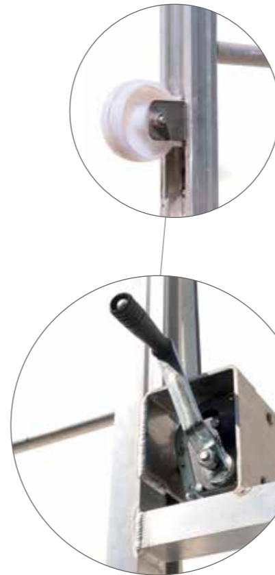
侧轮和手摇绞车
